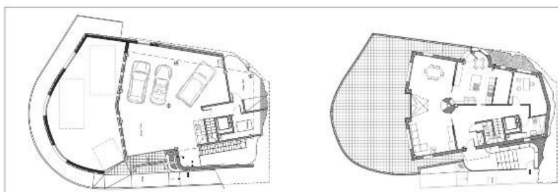
AMPLIACIÓ – PLANTA BAIXA
